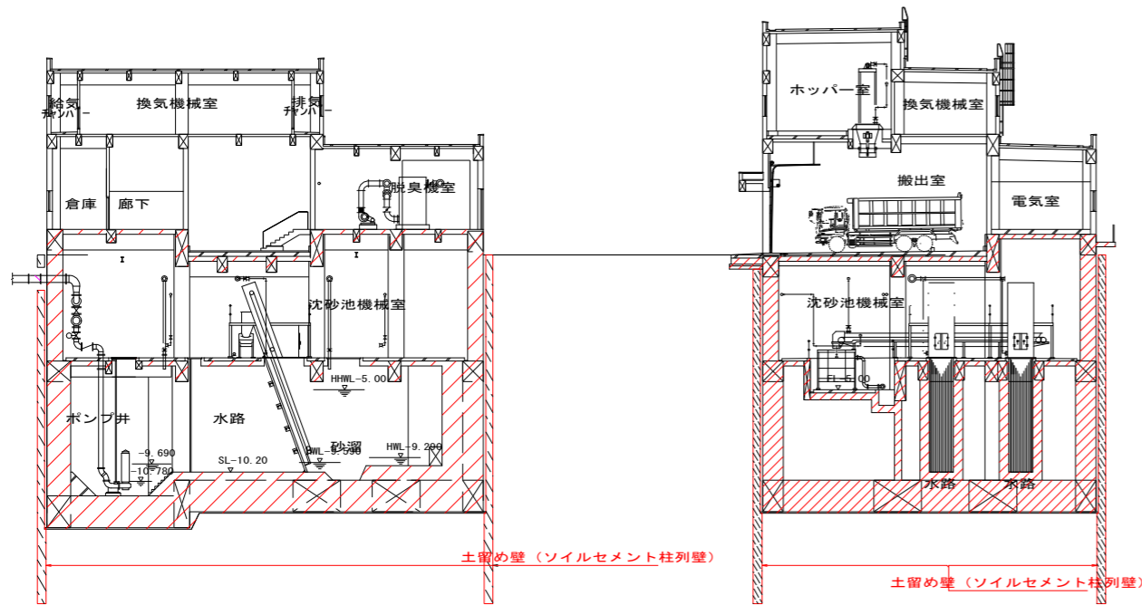
流入ポンプ棟 断面図
